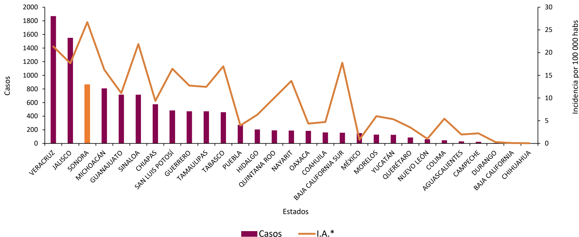
Casos confirmados de Dengue por entidad, SE 39 México 2025
